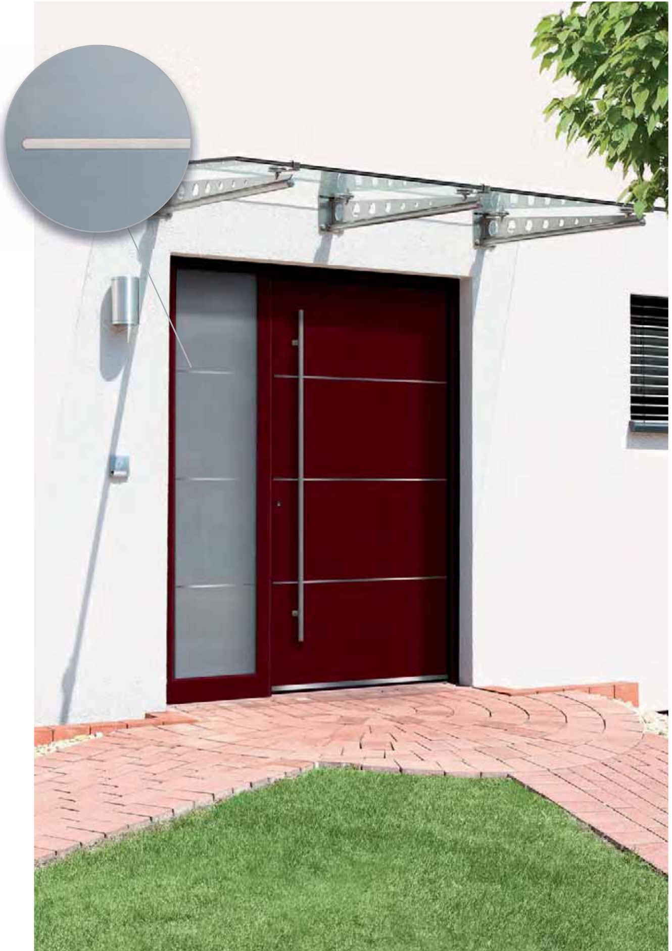
Modell 6872-94 flächenbündige Lisenen | Ganzglas-Seitenteil | Extras: Aufsatzfüllung | RAL 3005 weinrot | Designsockel SB 703-1 Glas Seitenteil: G 3001-94 Satinato weiß | Lisenen im Scheibenzwischenraum (auch erhältlich mit Klarglas) | Griff: 9028-13 Edelstahl, integriert
